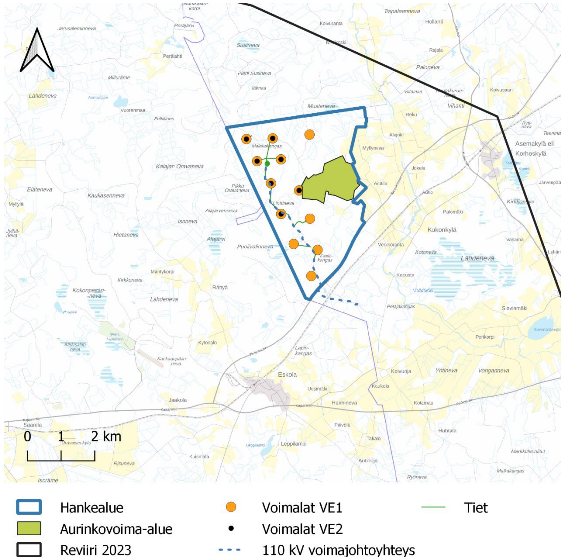
Kuva 4-1 Malakakankaan tuulivoimahanke YVA-menettelyn vaihtoehdot sekä Toholammin susireviirin sijainti vuonna 2023. Sähkönsiirto maakaapelilla hankealueen ulkopuolelle on kummassakin vaihtoehdossa sama.
